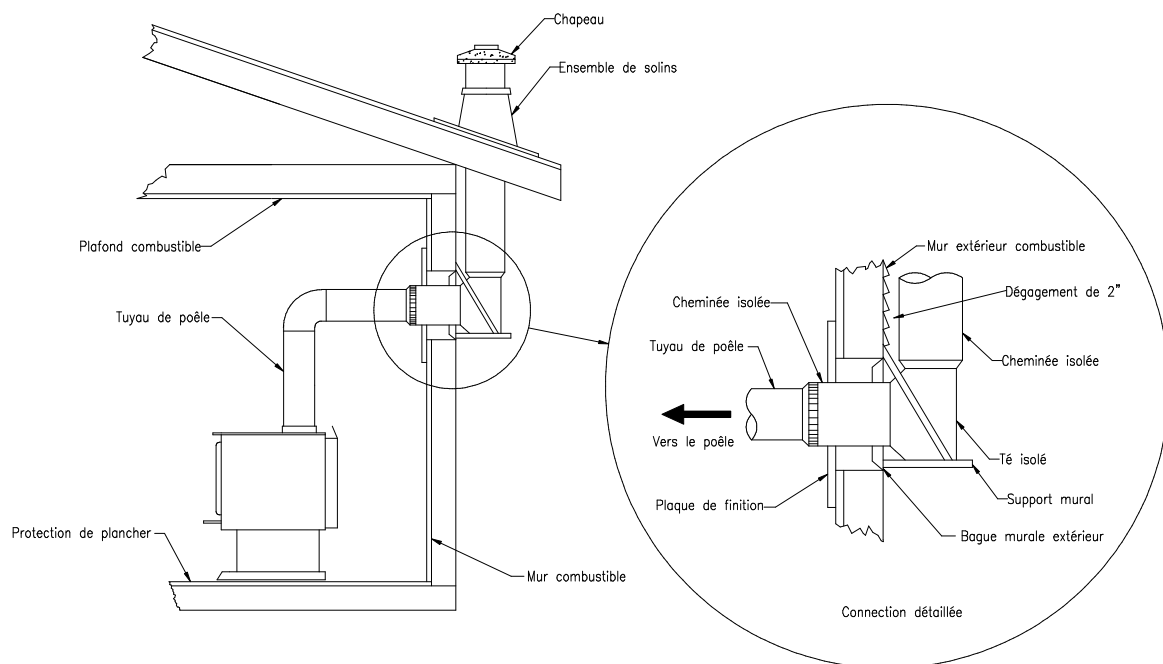
FIGURE 2.2.1 (A) Installation typique à travers le mur
